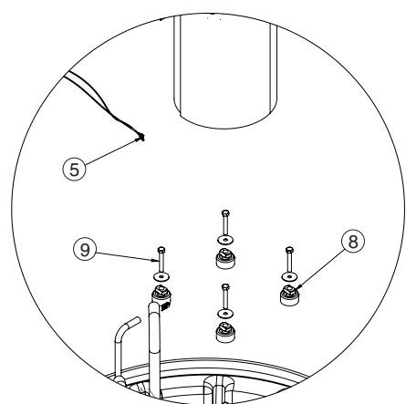
DÉTAIL C
