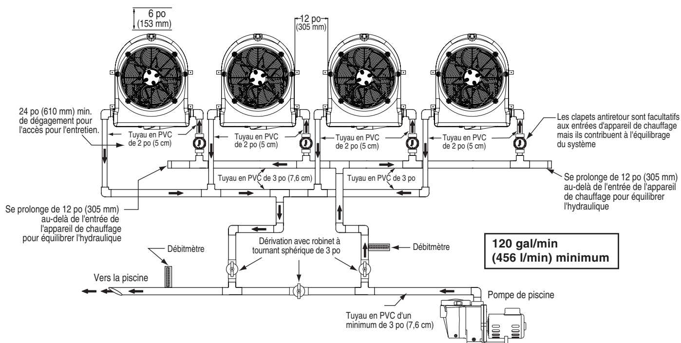
Disposition de la plomberie pour quatre thermopompes
