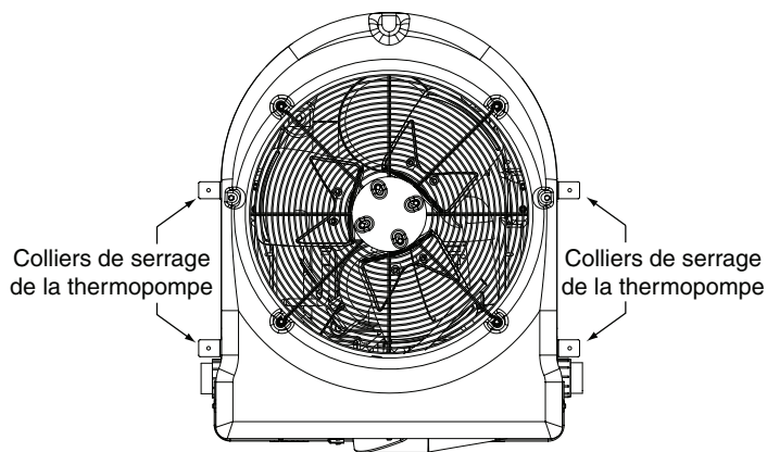
Installation des pinces d'ancrage
