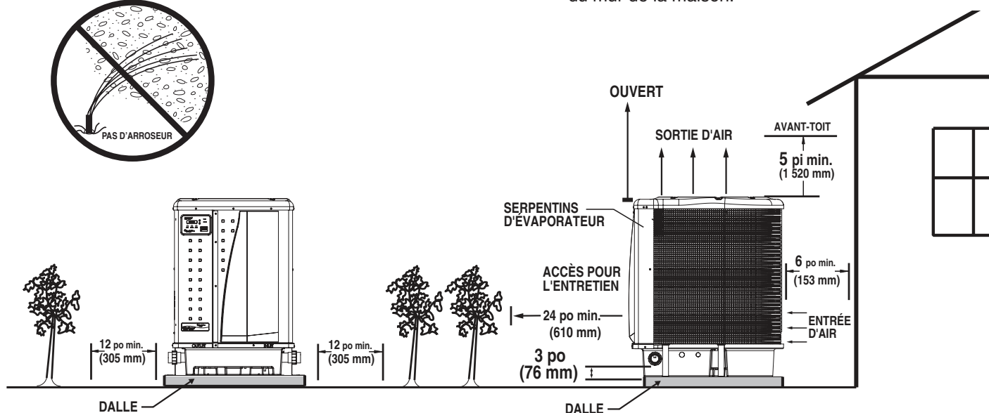
Emplacement de la thermopompe et dégagements
