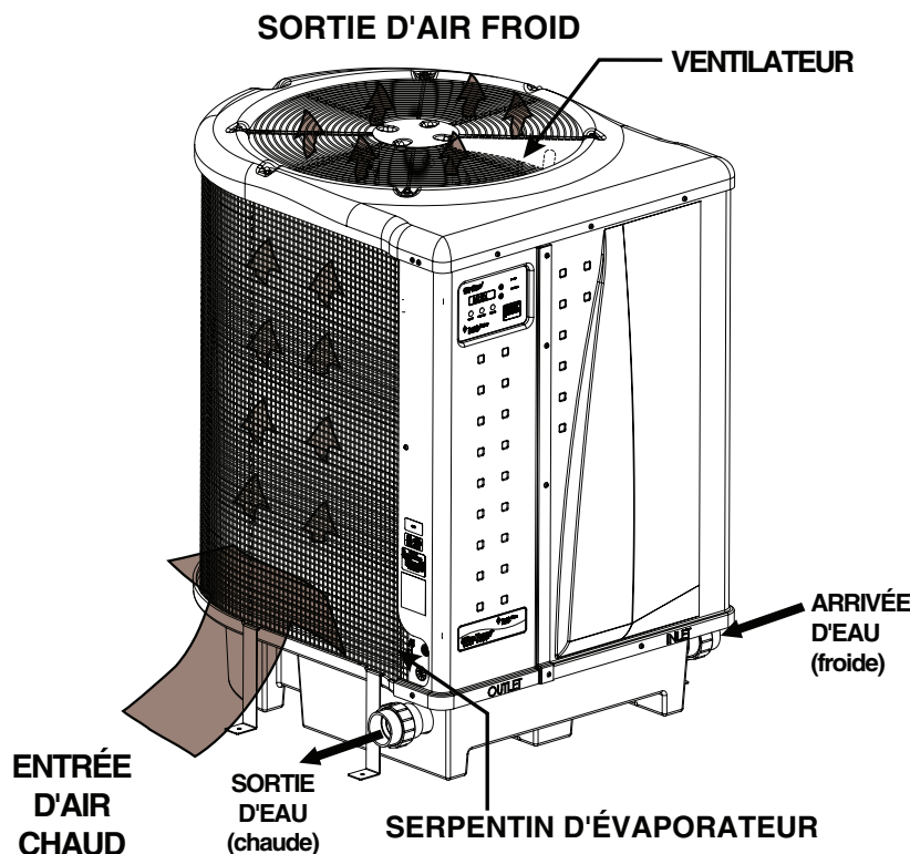
Cycle de chauffage type
