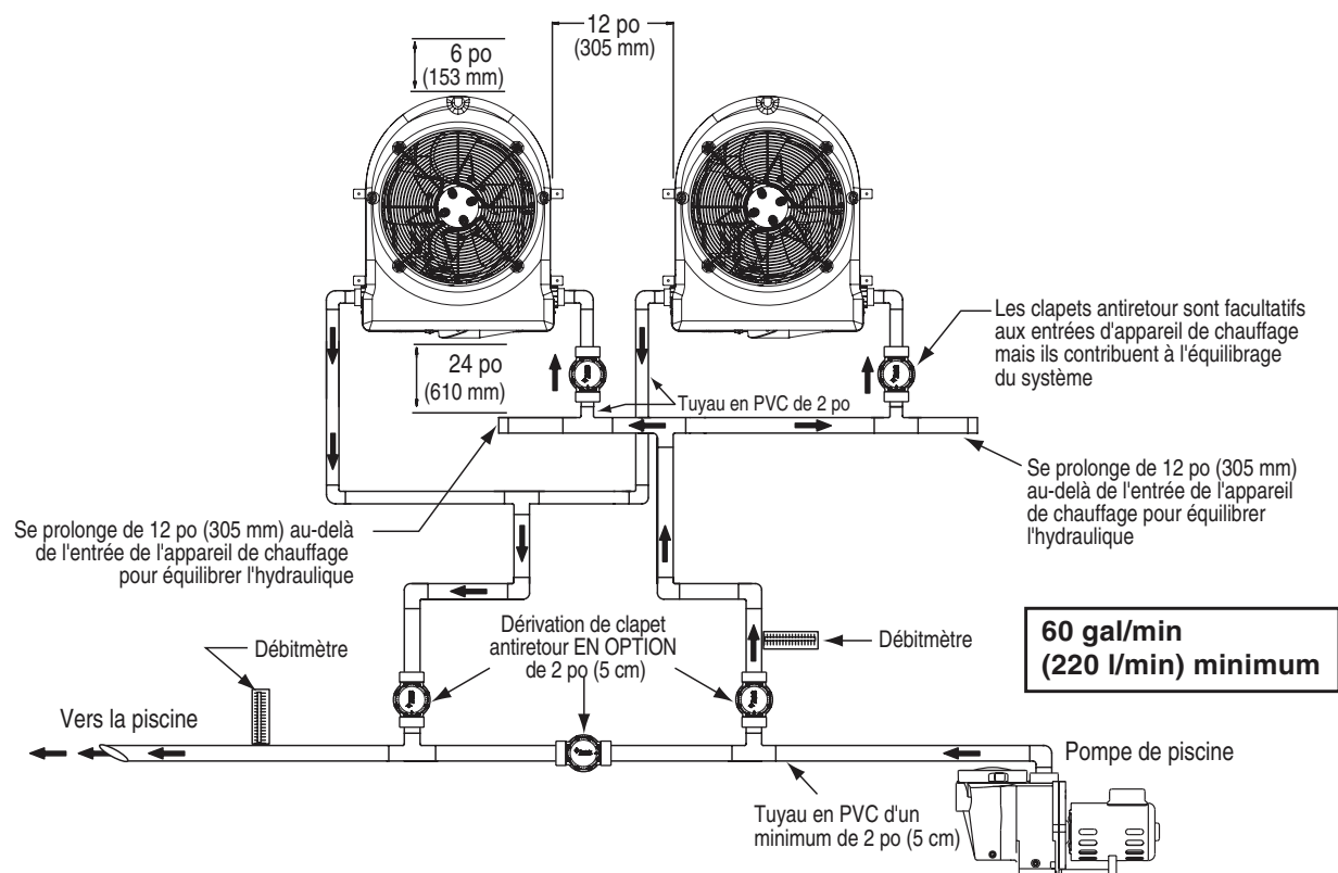
Disposition de la plomberie pour deux thermopompes
