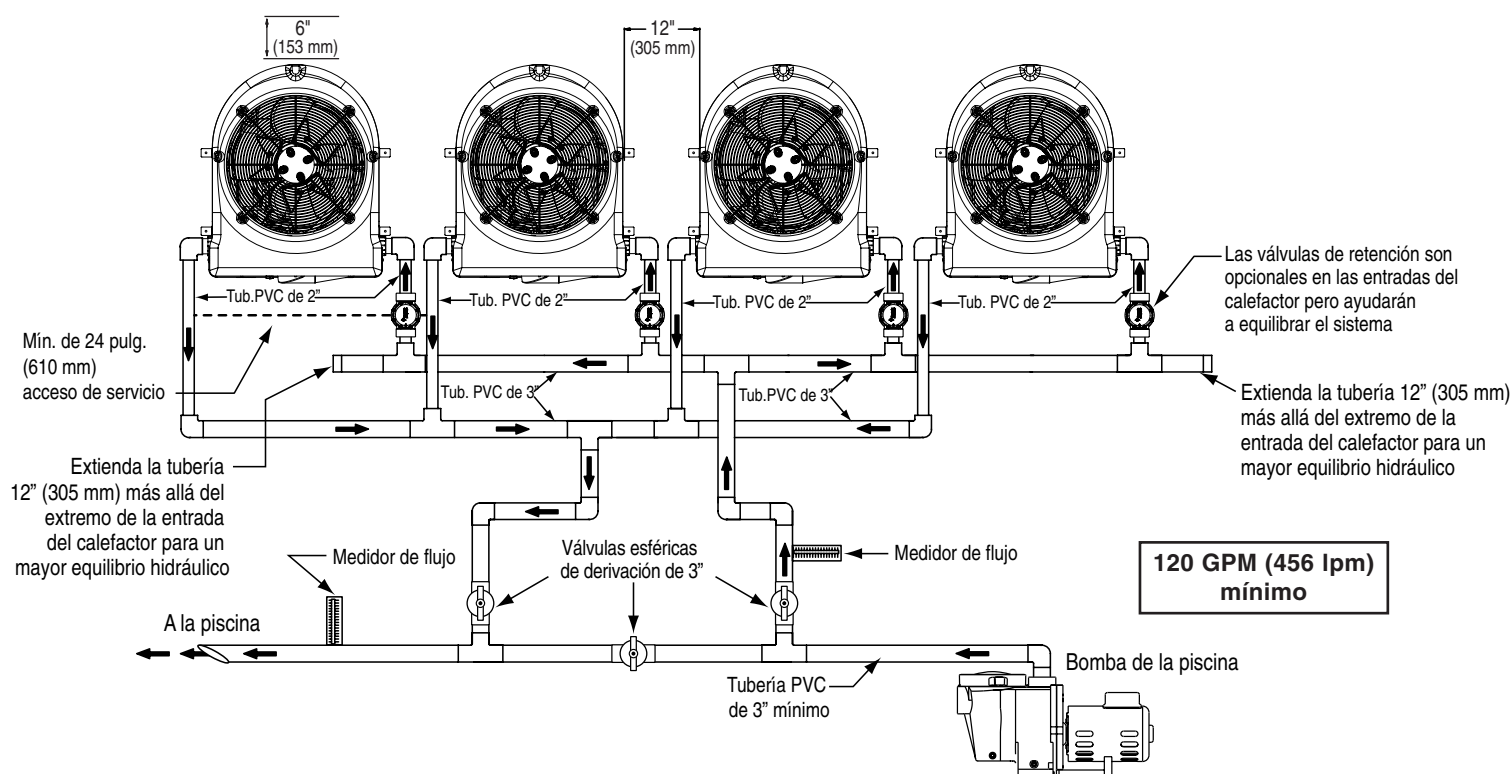
Disposición de las tuberías para cuatro bombas de calor
