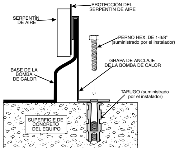
Instalación de grapa(s) de amarre
