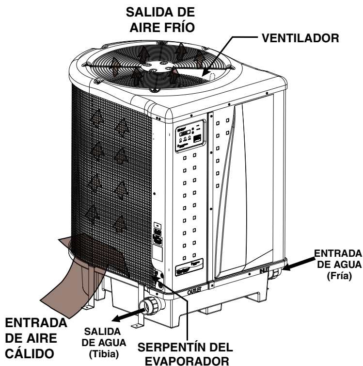
Ciclo típico de calentamiento
