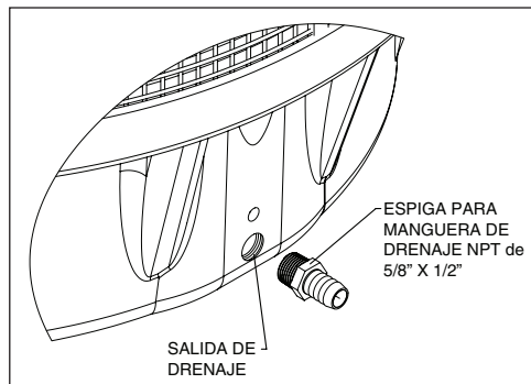
Instalación de la espiga para manguera de drenaje
