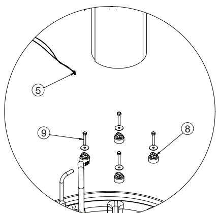
DETALLE C
