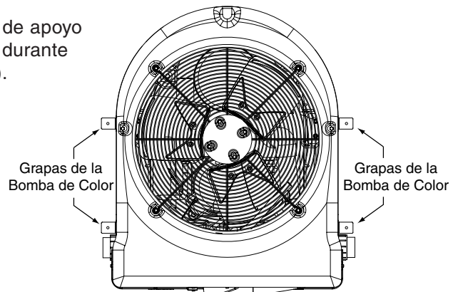
Instalación de grapa(s) de amarre
