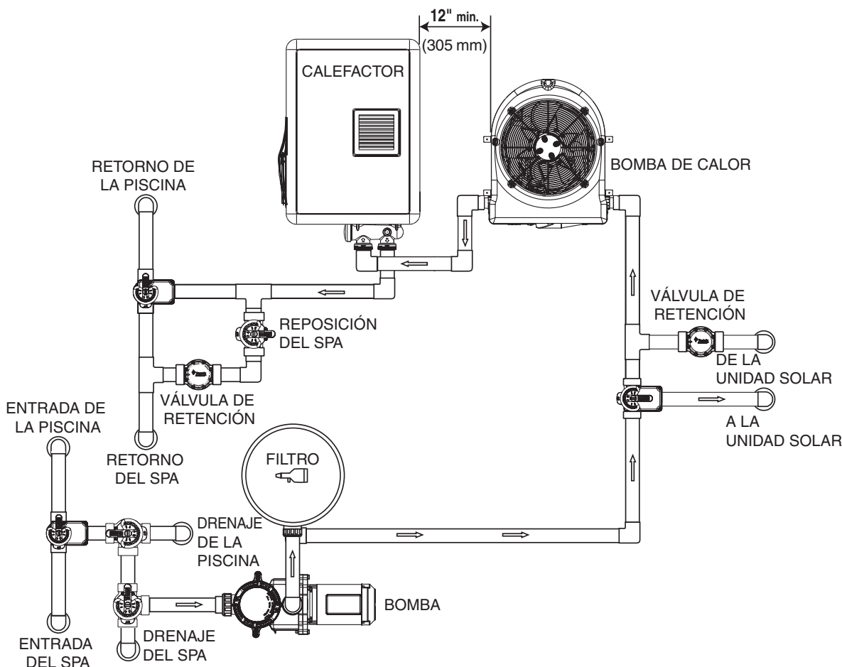
Instalación de varias unidades: Combinación de bomba de calor, calefactor
